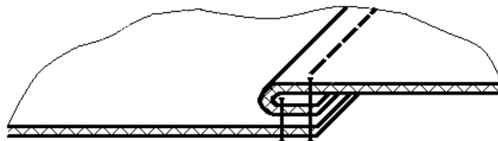
Настрочной шов
